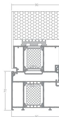
przekrój przez ościeżnicę i skrzydło, panel dwustronny, otwierany do wewnątrz
