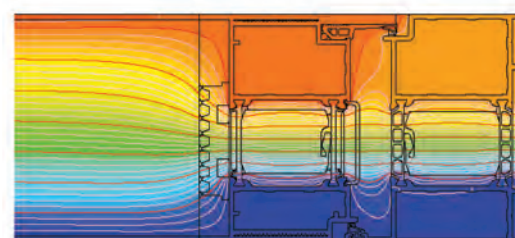
przykładowy rozkład izoterm dla złożeń ościeżnicy i skrzydła drzwi panelowych (GT 415 + GT 1626)
