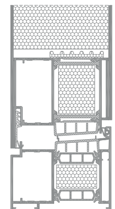
przekrój przez PD SP 800 i+
