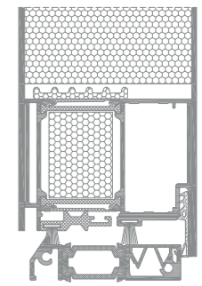
przekrój przez PD SP 800 i+
