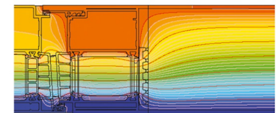
przykładowy rozkład izoterm dla systemu PD SP 800 i+
